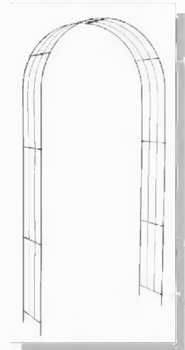
204-340-0200 Dim.: 114*34*246 cm
