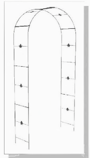
206-283-0100 Dim.: 114*34*226 cm
