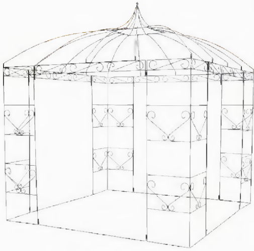
206-089-0100 Dim.: 240*240*300 cm
