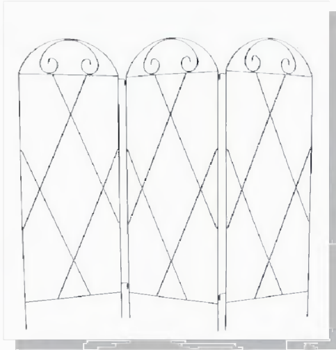
204-017-0100 Dim.: 175*2*160 cm
