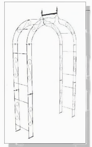
206-338-0200 Dim.: 139*39*240 cm
